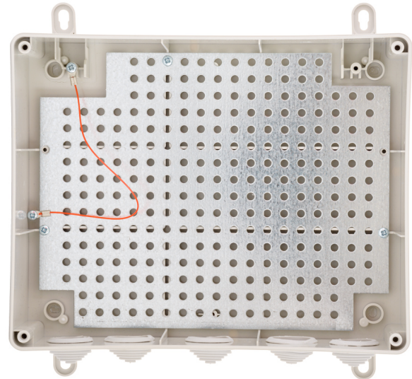
Przykład zabudowy blachy o obudowie ABOX-L3
