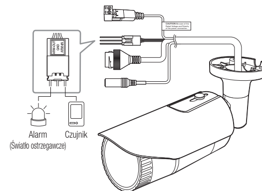
<QNV-7080R>
