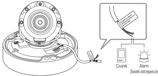
<QNV-7080R>
