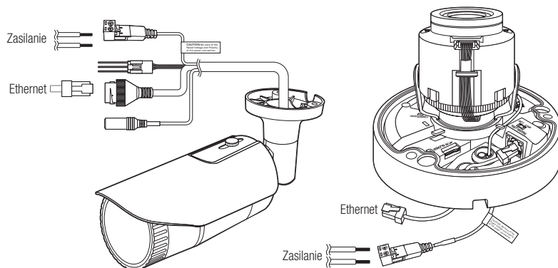
<QNO-7080R>
